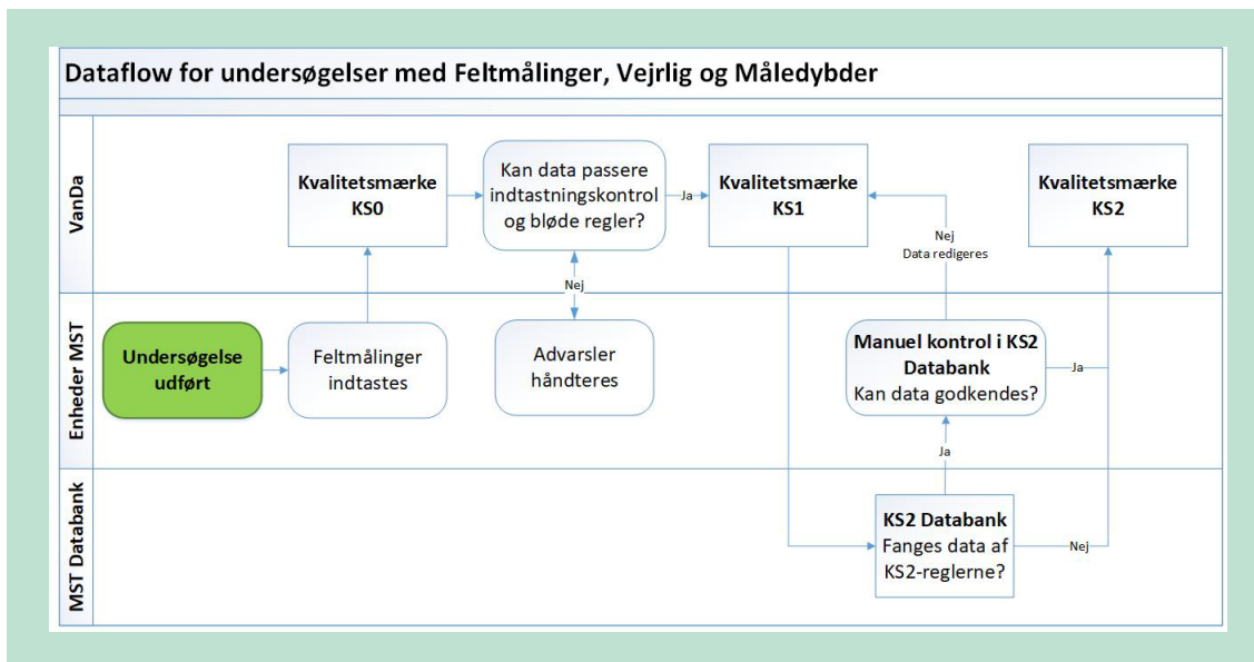
FIGUR 3. Dataflow for undersøgelsesemnerne Feltmålinger, Vejrlig og Måledybder som indtastes direkte i VanDa. Flowet starter ved den grønne boks "Undersøgelse udført" og læses fra venstre mod højre.
