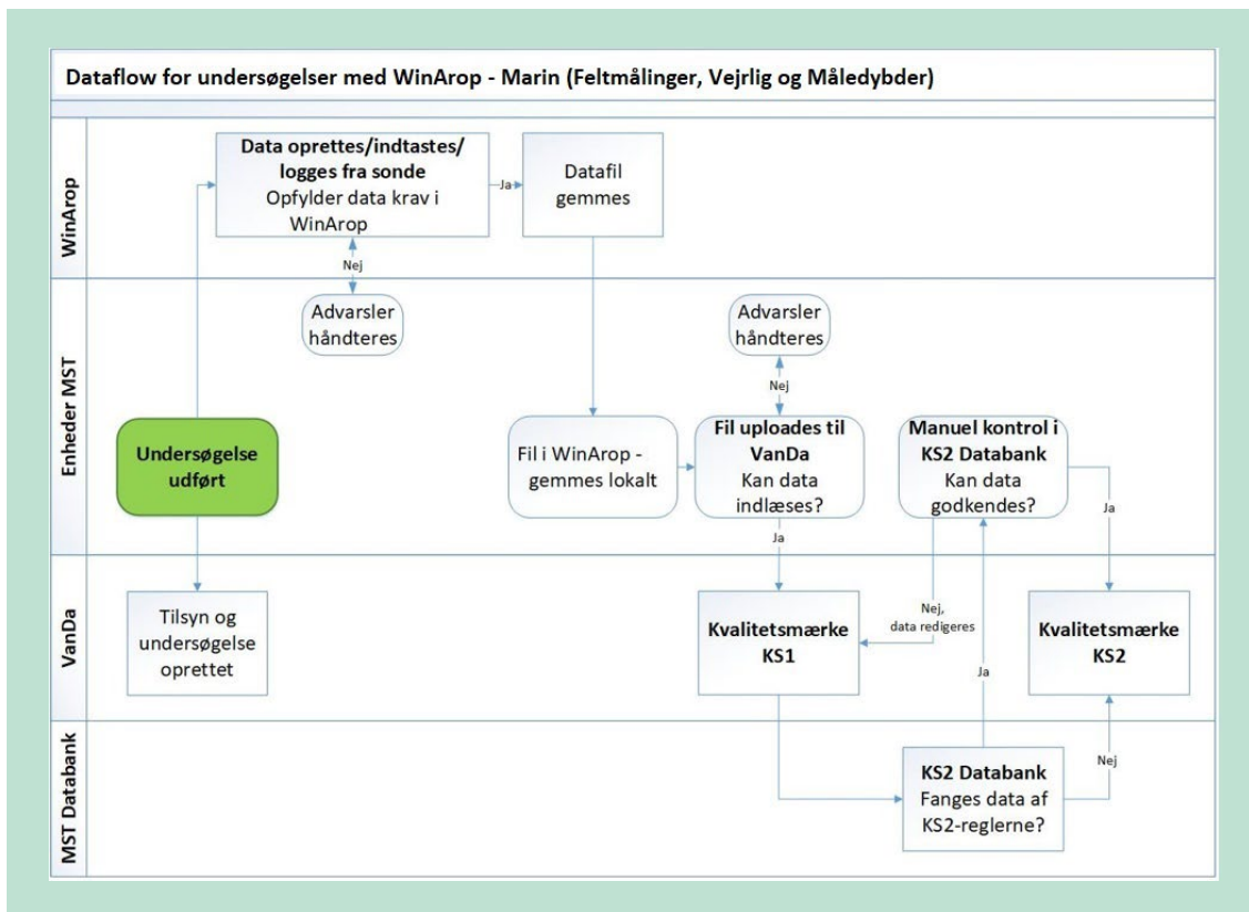
FIGUR 2. Dataflow for Feltmålinger opsamlet ved brug af WinArop. Flowet starter ved den grønne boks "Undersøgelse udført" og læses fra venstre mod højre.
