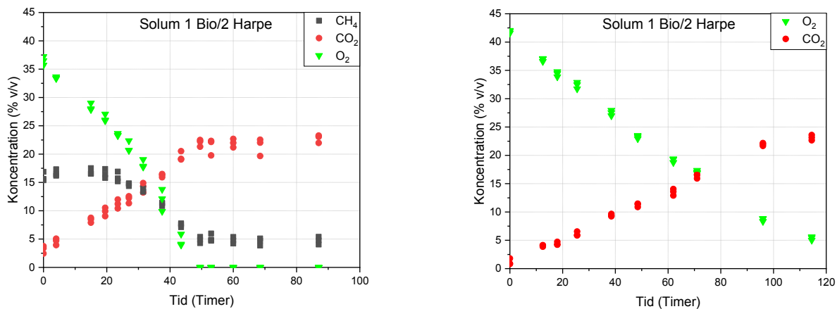
Figur 1. Udviklingen af gaskoncentrationer målt i headspace over tid i batchforsøg. I metanoxiderationsforsøgene blev der målt \text{CH}_4 , \text{CO}_2 og \text{O}_2 (tv), mens der i respirationsforsøgene blev målt \text{CO}_2 og \text{O}_2 (th). For hvert måletidspunkt er der tre punkter tilhørende hvert batchforsøg, idet de blev udført som triplikater.
