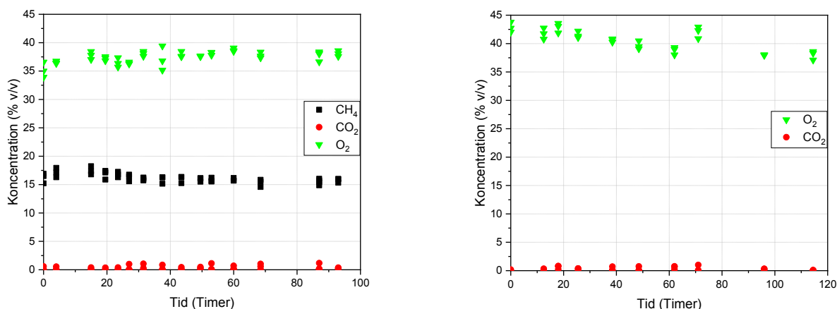
Figur 2. Udviklingen af gaskoncentrationer over tid i kontrolforsøg. I metanoxiderationsforsøgene blev der målt CH 4 , CO 2 og O 2 (tv), mens der i respirationsforsøgene blev målt CO 2 og O 2 (th). For hver gas er der tre punkter tilhørende hver måling, da forsøgene blev udført i triplikater.
