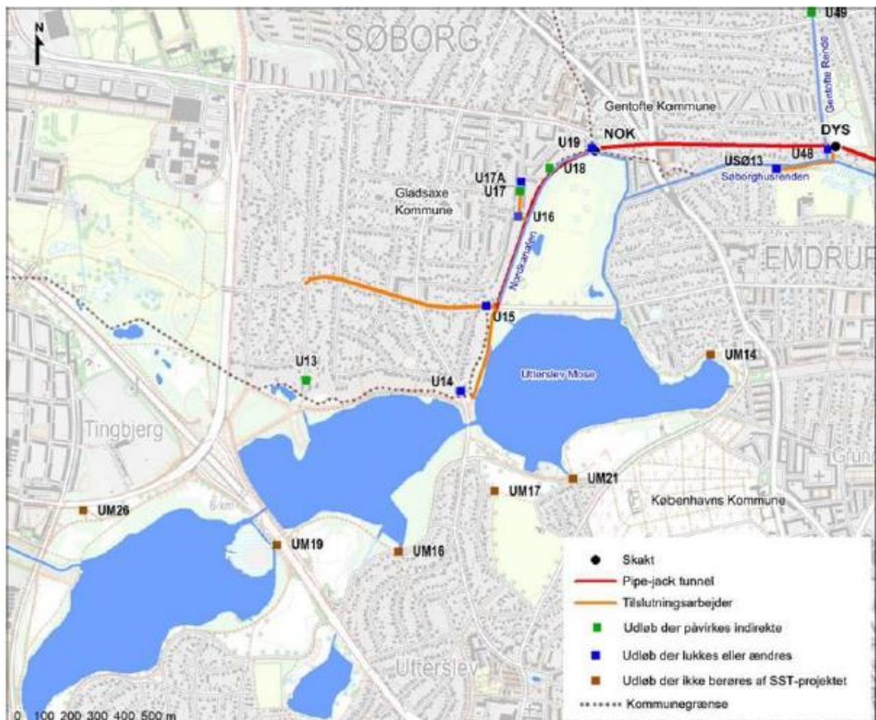
Figur - - Oversigt over Utterslev Mose, Nordkanalen, Gentofterenden og Søbørghusrenden samt udledningspunkterne til disse vandområder. De blå og grønne udløb påvirkes af Svanemøllen Skybrudstunnel.
