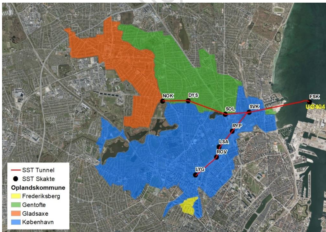
Figur 2- Udledningspunkt UØ404 til Øresund på Fiskerihavnen (FSK) samt overløbsoplandet.
