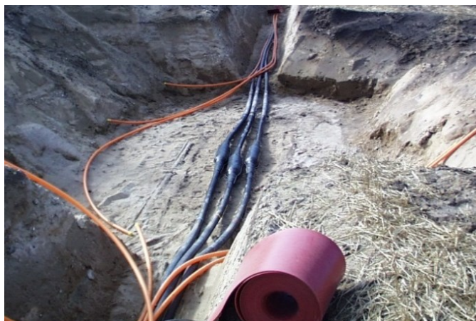
Figur 2-32 Kablerne er muffet sammen
