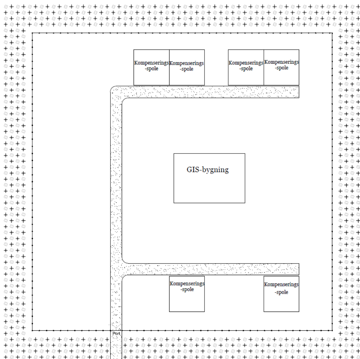
Figur 5-2 Oversigtstegning over kompenseringsstation.
