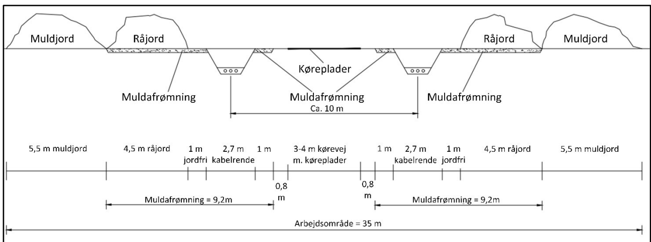
Figur 2-1 Princip for tværsnit af anlægsbælte til to 275 kV kabelsystemer
