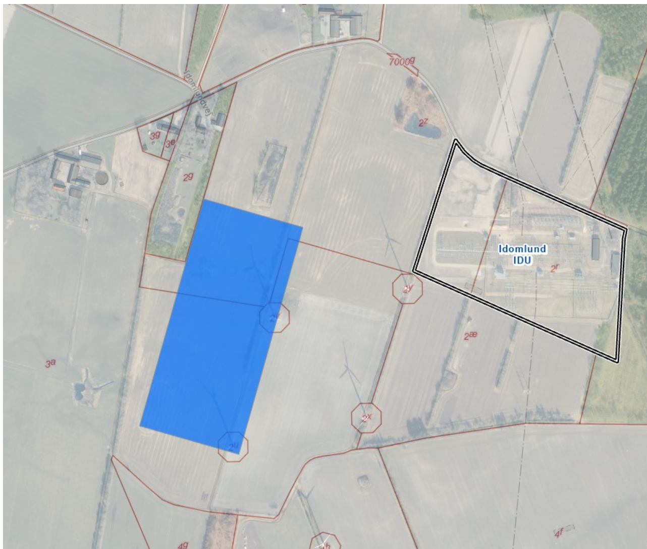
Figur 4-4. Den nye koblingsstation placeres vest for den eksisterende station Idomlund i Holstebro Kommune og tilkobles denne. Arealet til stationen udgør ca. 7,2 ha (400x180m).
