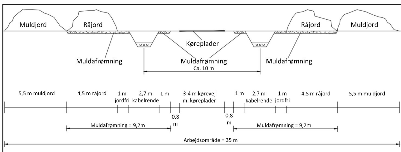
Figur 2-1. Princip for tværsnit af anlægsbælte til to 220 kV kabelsystemer
