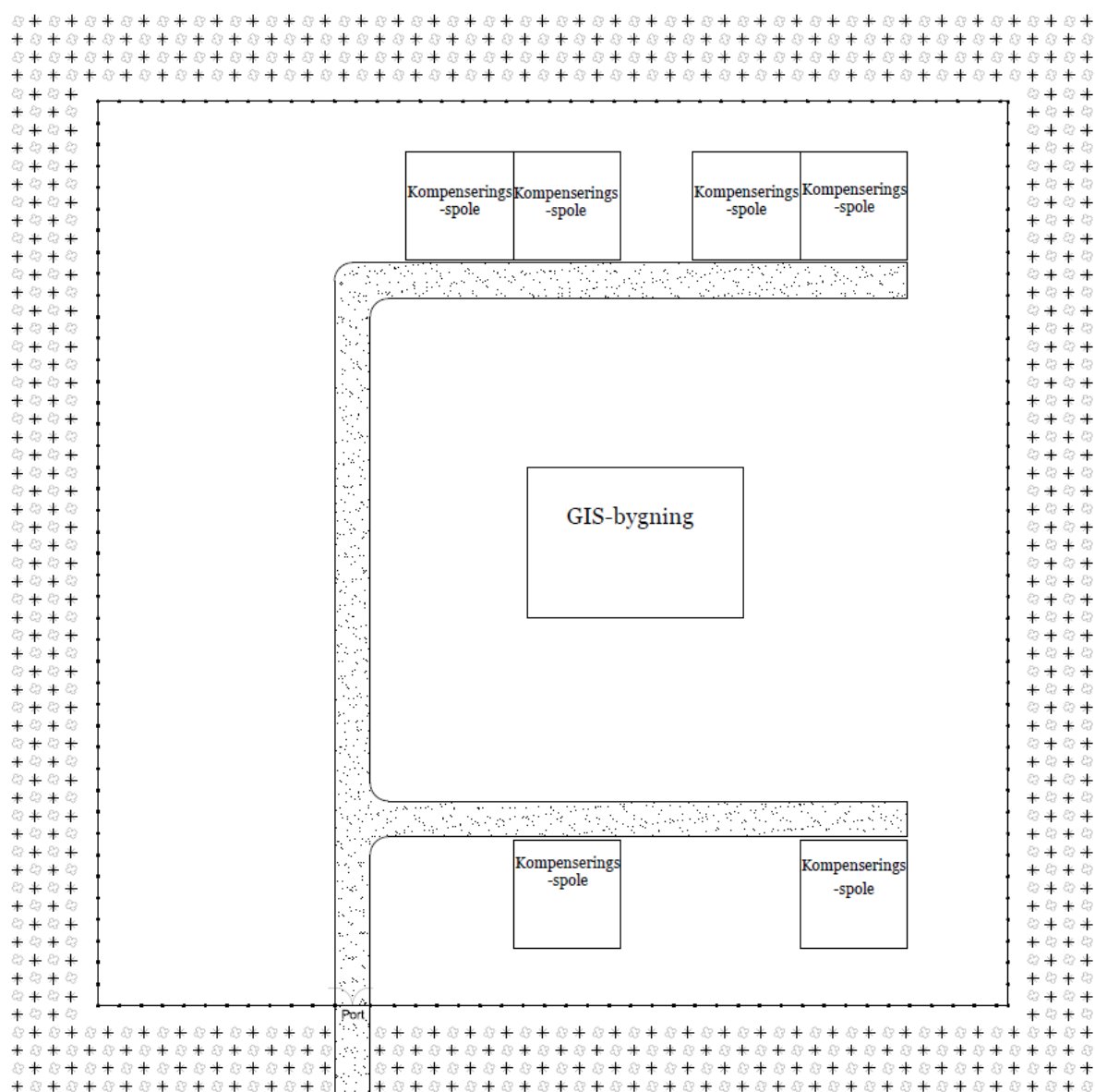
Figur 4-2 Oversigtstegning over kompenseringsstation.
