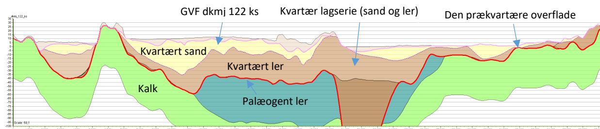
Figur 1: Udvalgt V-Ø profil gennem GVF dkmj 122 ks (hydrostratigrafisk model) /1/.
