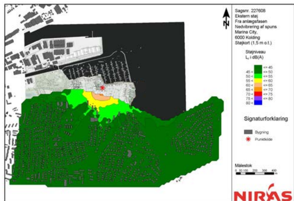
Figur 7-6: Støj fra nedvibrering af spuns/pilotering.
