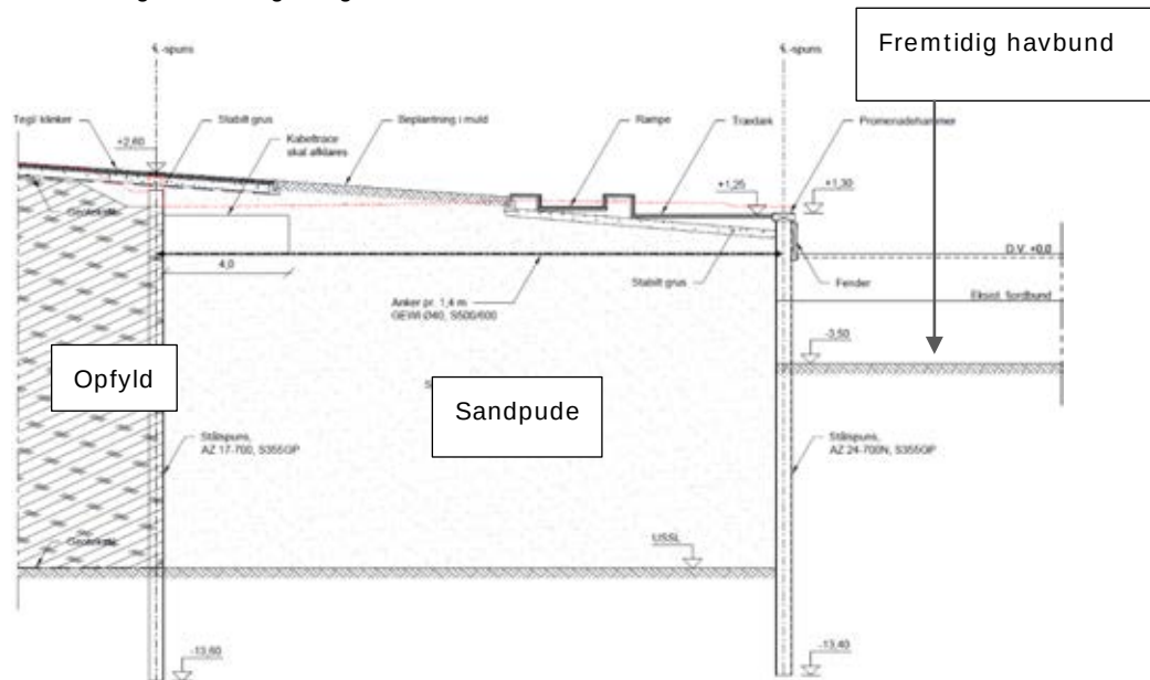
Figur 3-31: Opbygning af spunsvæg ud for opfyldningsområde vest. Snittet kan ses i større format i bilag 5.
