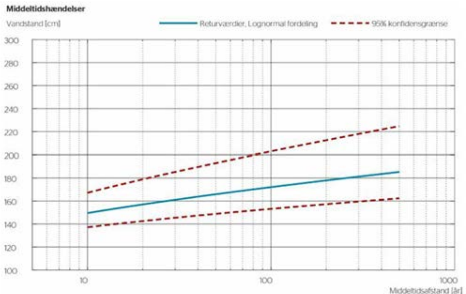
Figur 10-1: Højvandsstatistik 2017 for Kolding Havn (Kystdirektoratet, 2018).
