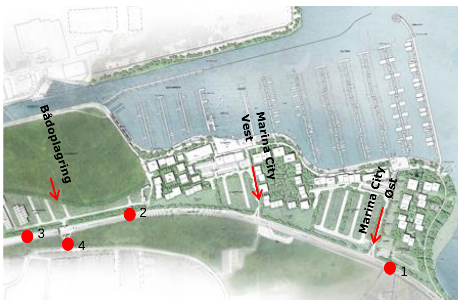
Figur 9-4: Trafiktællepunkter og udkørsler til Skamlingvejen på baggrund af illustrationsplan for Marina City.
