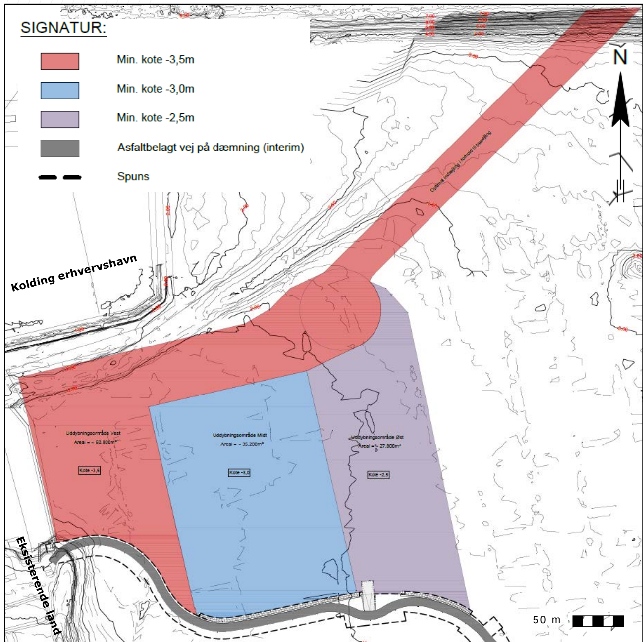
Figur 3-3: Uddybning af udvidet havnebassin og sejlrunde sker i røde, blå og lilla områder. Se også skitse i større format i bilag 5.
