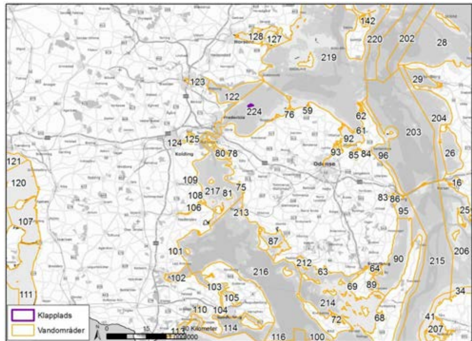
Figur 16-2: Vandområder omkring Trelde Næs klappblads jævnfør vandområdeplanen for 2015-2021. Trelde Næs klappblads er markeret med en lilla firkant i vandområde 224 (Vejdirektoratet, 2016).
