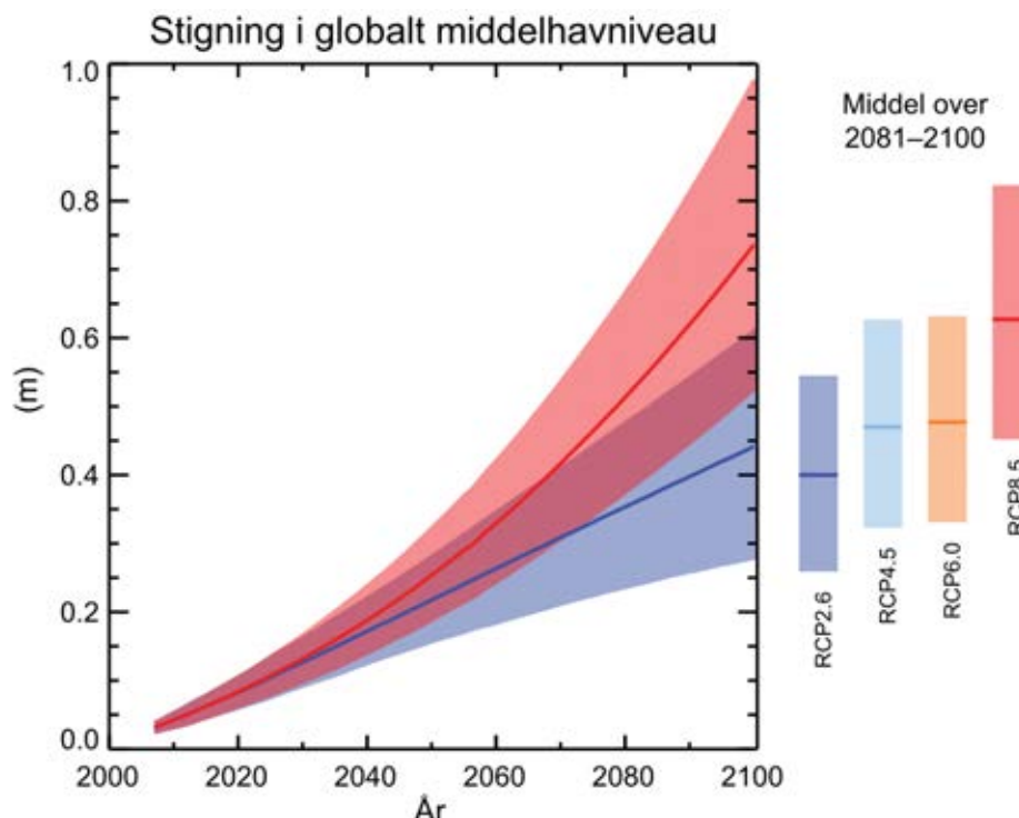
Figur 10-3: Stigning i globalt middelhavniveau, ved 2 (4) klimascenarier (Klimatilpasning.dk, 2014).
